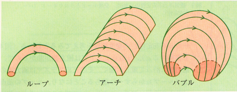
図2 磁気ループ、アーチ、バブル。
