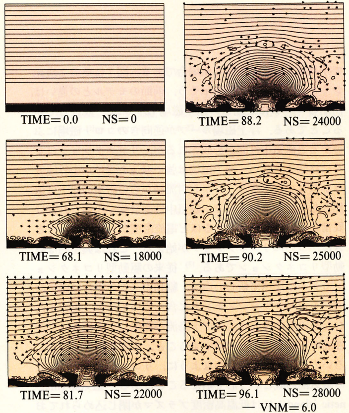
図7 浮上磁場にもなるリコネクション。磁力線と速度場の時間発展を示す。初期のコロナには浮上磁場と逆向きの水平磁場 ( \beta=0.2 ) がある。計算領域、長さ、時間の単位などは、図6のケースと同じ。複数の磁気島が融合しながら中性面に沿って噴出していることに注意。
