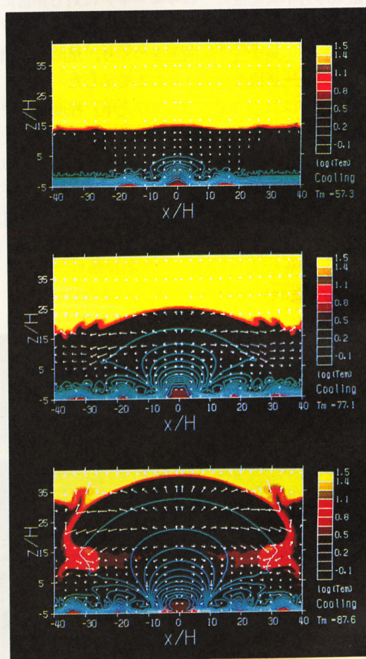
図6 浮上磁場の2次元 MHD モデル (野沢, 松元, 柴田, 諸氏よりの提供)。図は温度分布と磁力線分布を示す。計算領域は上からコロナ (温度分布で黄色のところ)、彩層, 光球, 対流層 ( z < 0 の領域) となっており、対流層に初期条件として水平な孤立磁束 ( \beta = 4 ) が埋め込まれている。初期の彩層とコロナには磁場はない。長さの単位はスケールハイト \Lambda (図中では H と表示されている) で、太陽表面では約 200 km に対応する。時刻 t/\tau = 57.3, 77.1, 87.6 における図が示されている。ただし、時間の単位は \tau = \Lambda / C_0 \approx 20 秒。下降流による衝撃波加熱によって数万度の高温領域 (ループ足元の赤いところ) ができていることに注意。下降流の最大値は約 50 \text{ km s}^{-1} 。磁気ループは上昇するにつれて低 \beta ( \sim 0.01-0.1 ) ループに進化する。
