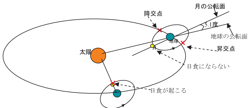
図2. 昇交点か降交点で新月となれば日食が起こる
