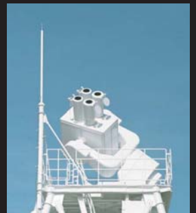
最新型の4連式望遠鏡 「SMART」(飛騨天文台)
