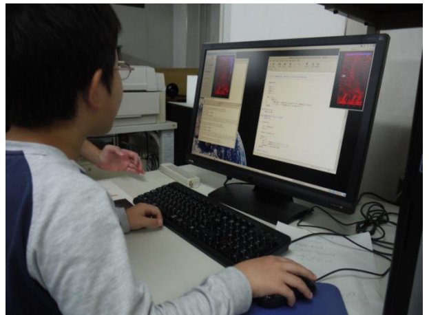
コンピューターを使った天文学研究体験コーナー
