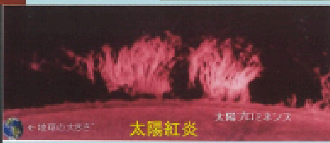
水素H \alpha 線で見た太陽像
