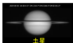
土星
