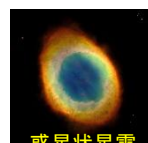
惑星状星雲
