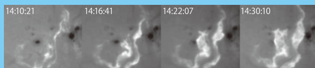
18cm 屈折望遠鏡で観測した 2001 年 4 月 10 日の太陽フレア
