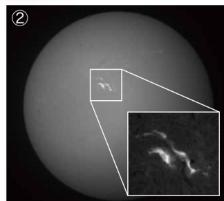
〈左〉①太陽プロミネンス（2022年9月15日）〈右〉②中規模フレア（2021年11月2日） 別館：18cm屈折ザートリウス望遠鏡。晴天時には、リアルタイムの太陽画像を観察できます。
